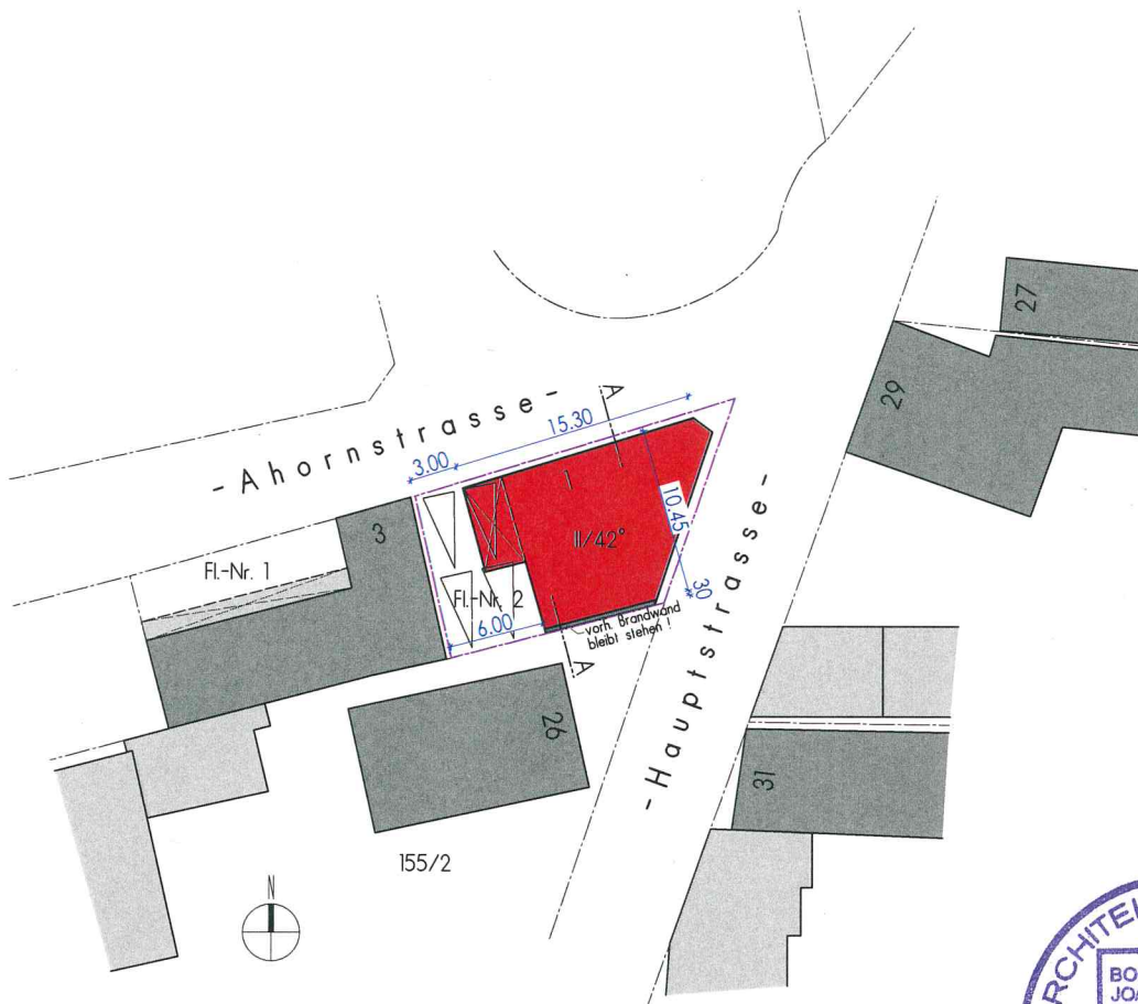
Lageplan M. 1:500
