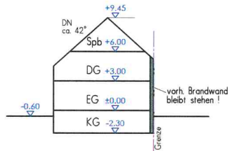
Schnitt A-A
