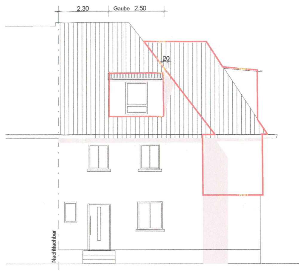
OSTANSICHT
