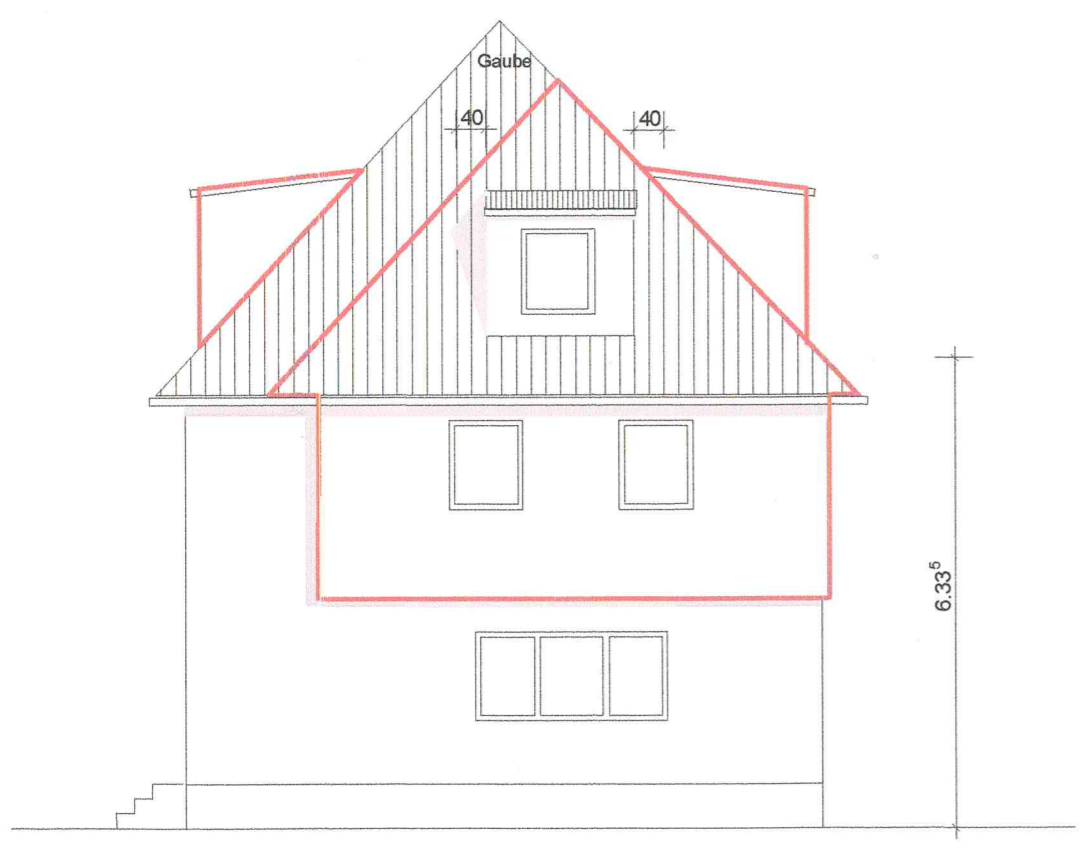
NORDANSICHT
