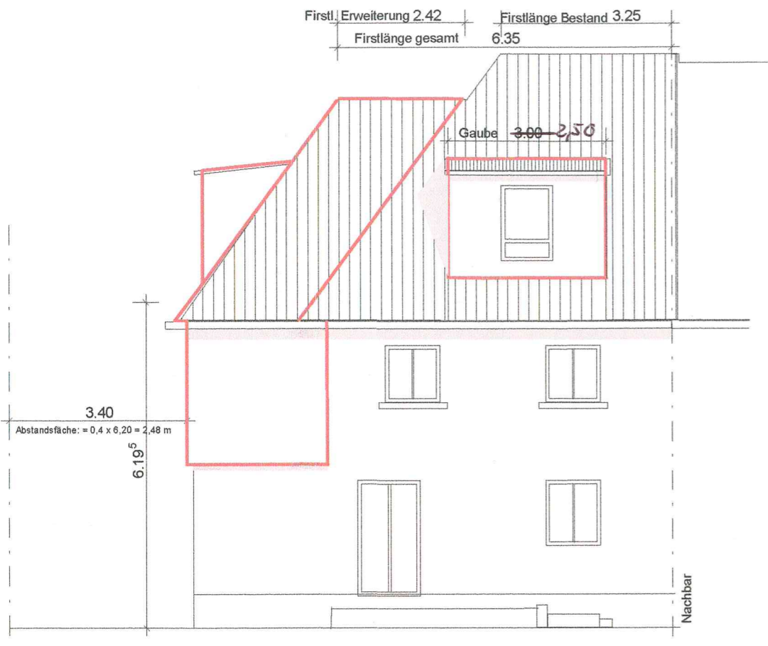
WESTANSICHT
