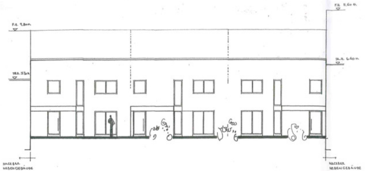
WEST-ANSICHT
