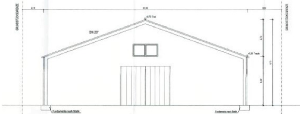
Schnitt A-A
