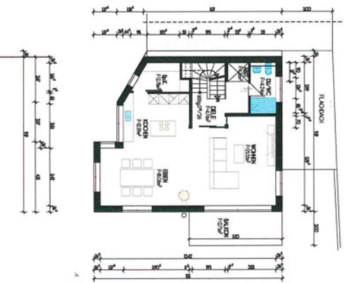
GRUNDRISS OBERGESCHOSS
