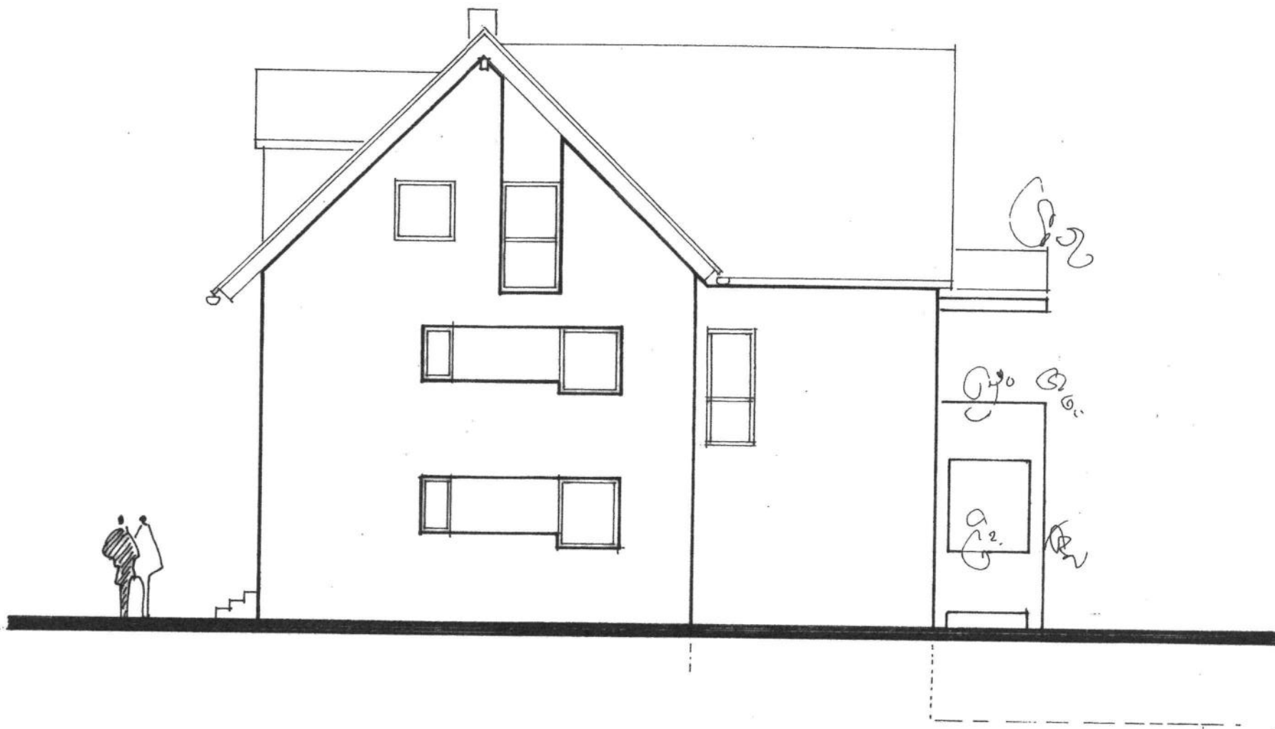
N O R D - A N S I C H T W O H N H A U S N R. 10
