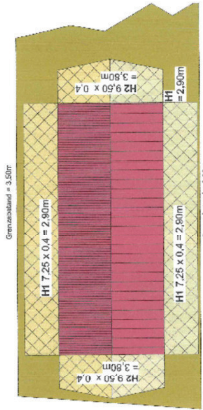
Abstandsflächen M. 1:200
