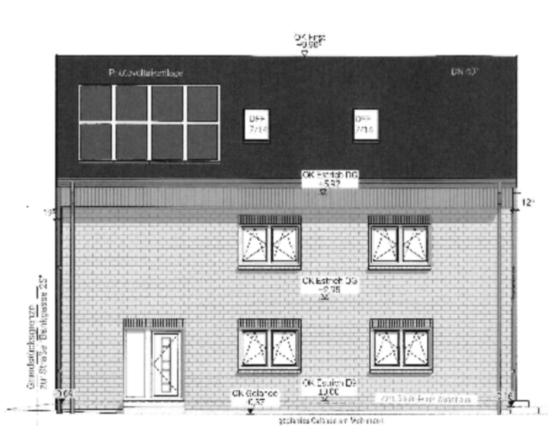
Ansicht 1
