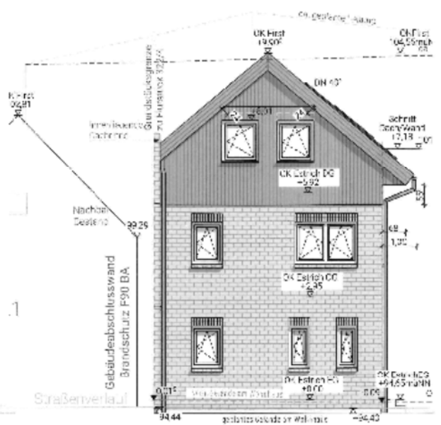
Ansicht 2
