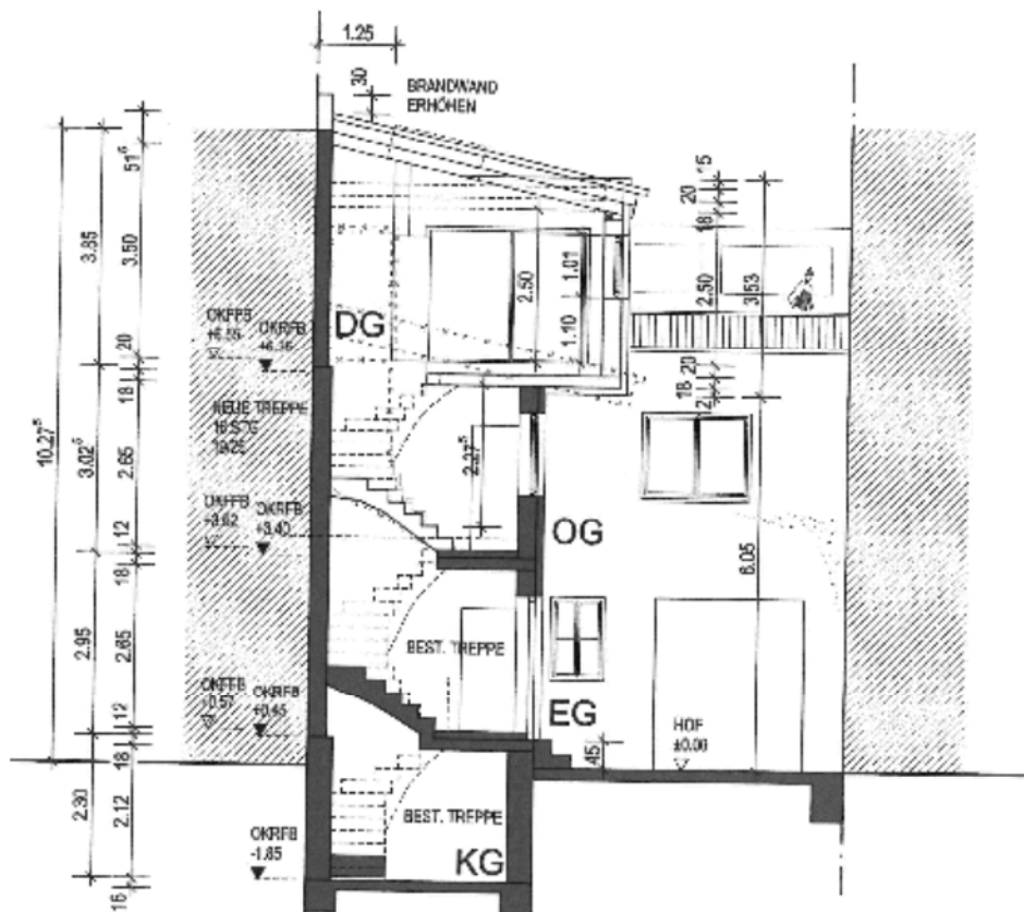
SCHNITT B-B
