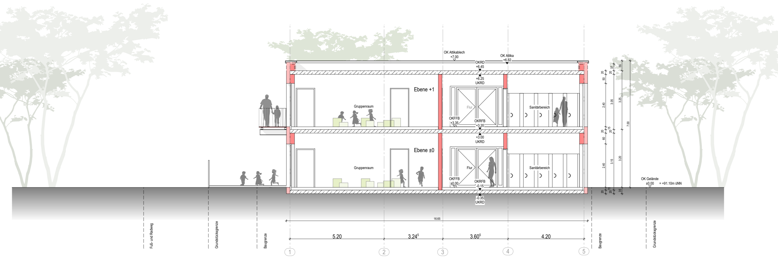
Gebäude B_Schnitt D
