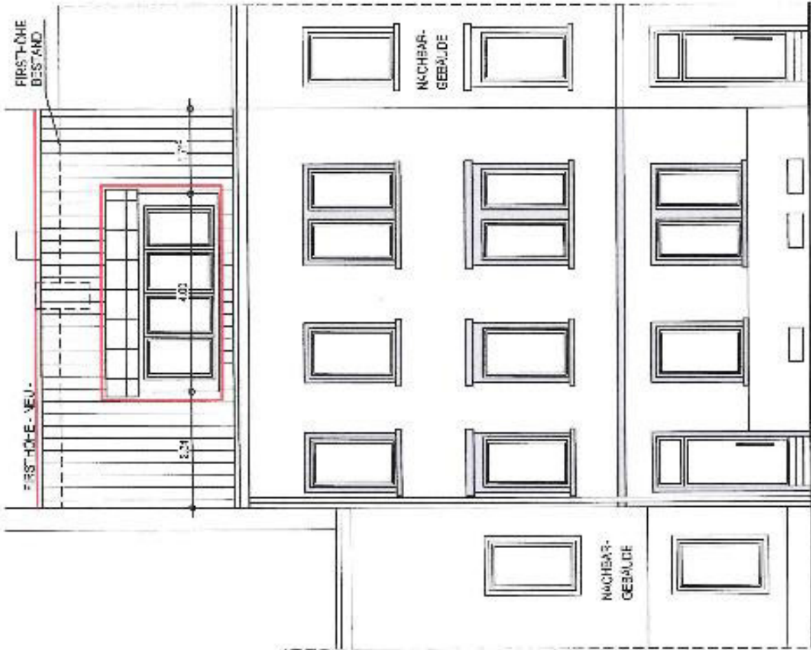
ANSICHT SÜDEN WILLESTRASSE
