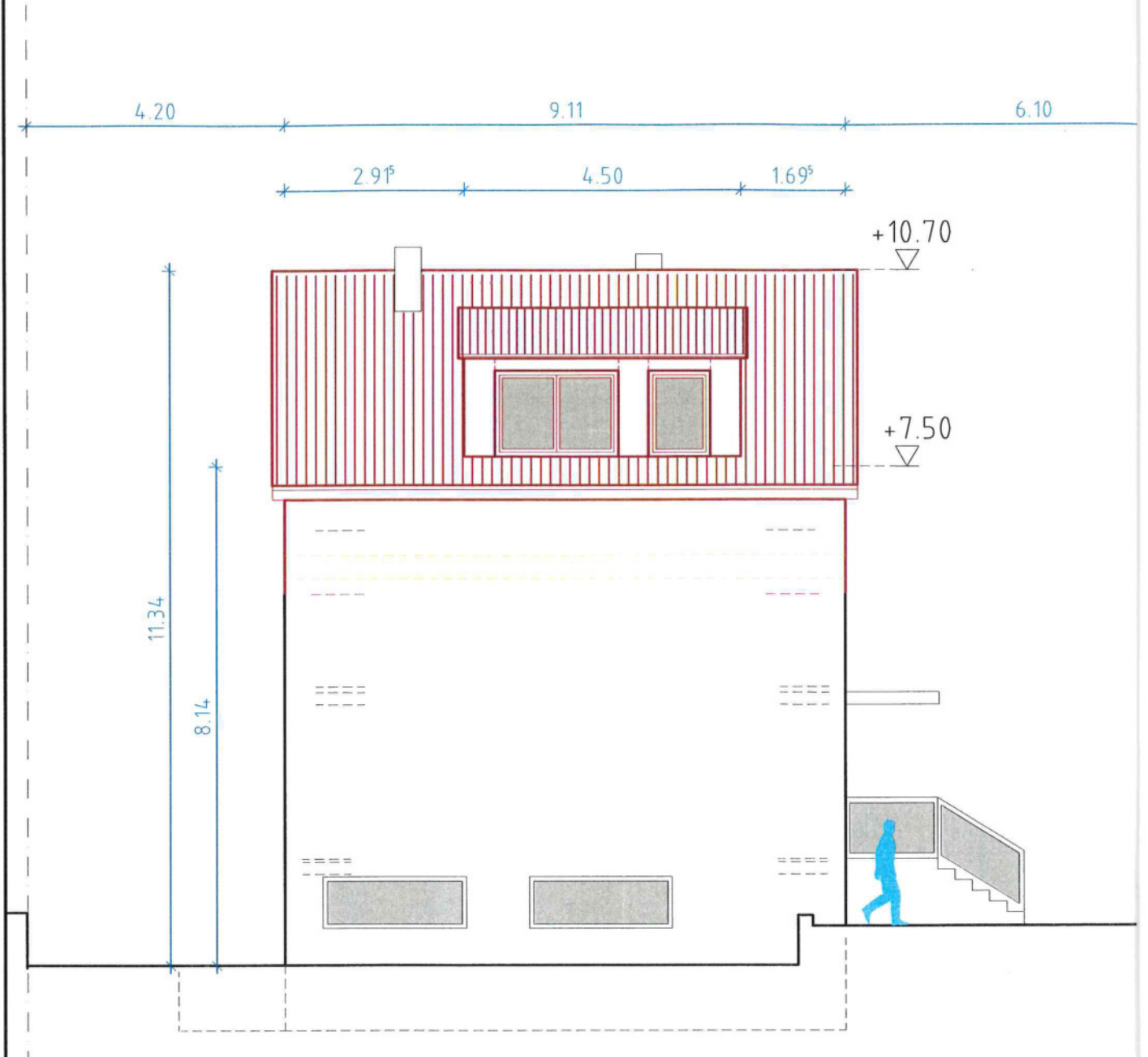
SÜDANSICHT M=1:100
