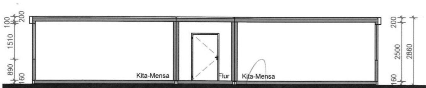
SCHNITT
