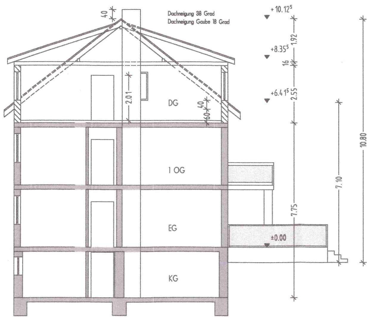
SCHNITT A-A
