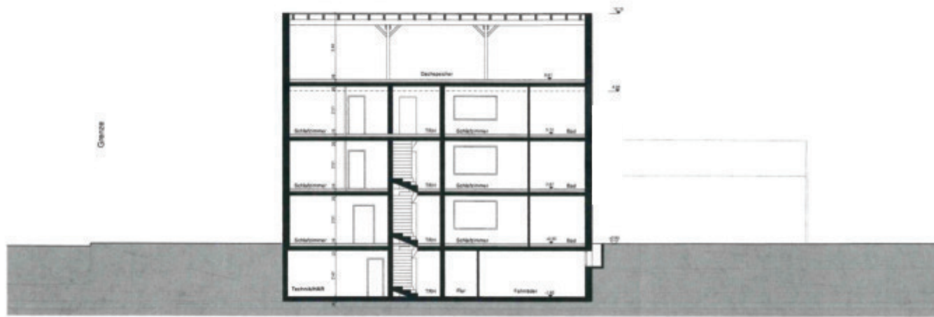
Schnitt S01
