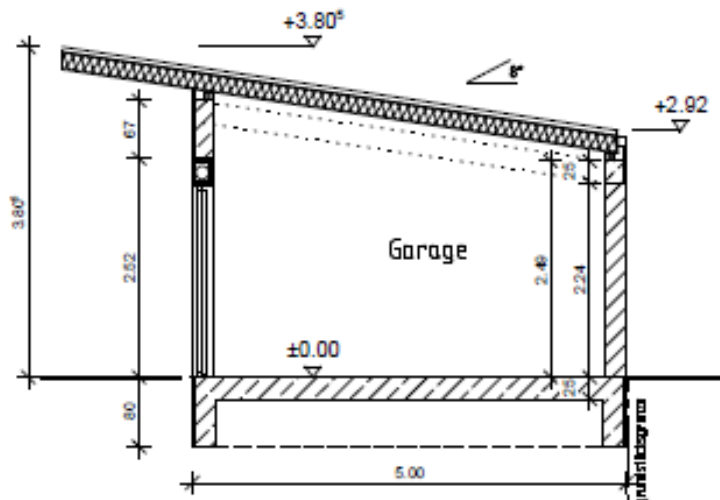
Schnitt A-A
