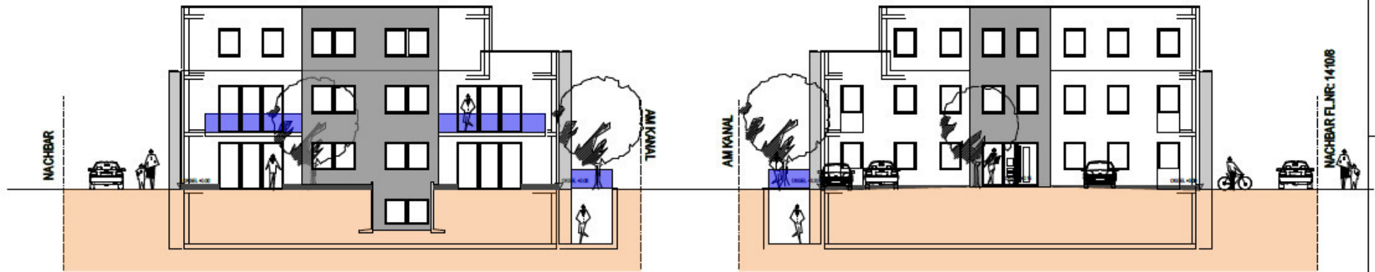
ANSICHT VON WESTEN
