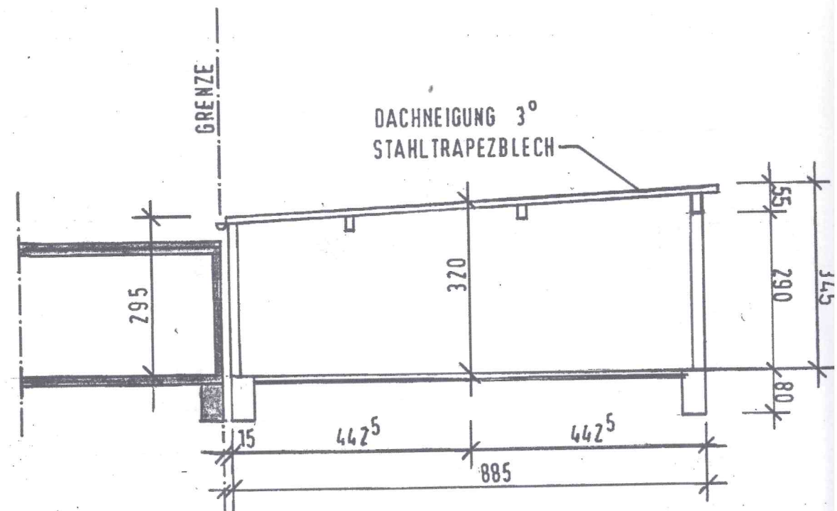
SCHNITT GARAGE
