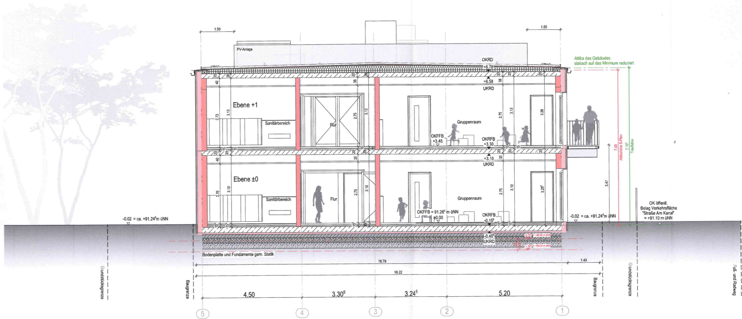
Gebäude A_Schnitt D
