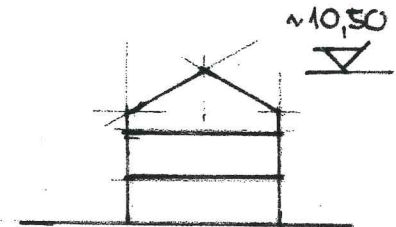
SCHNITT B-B
