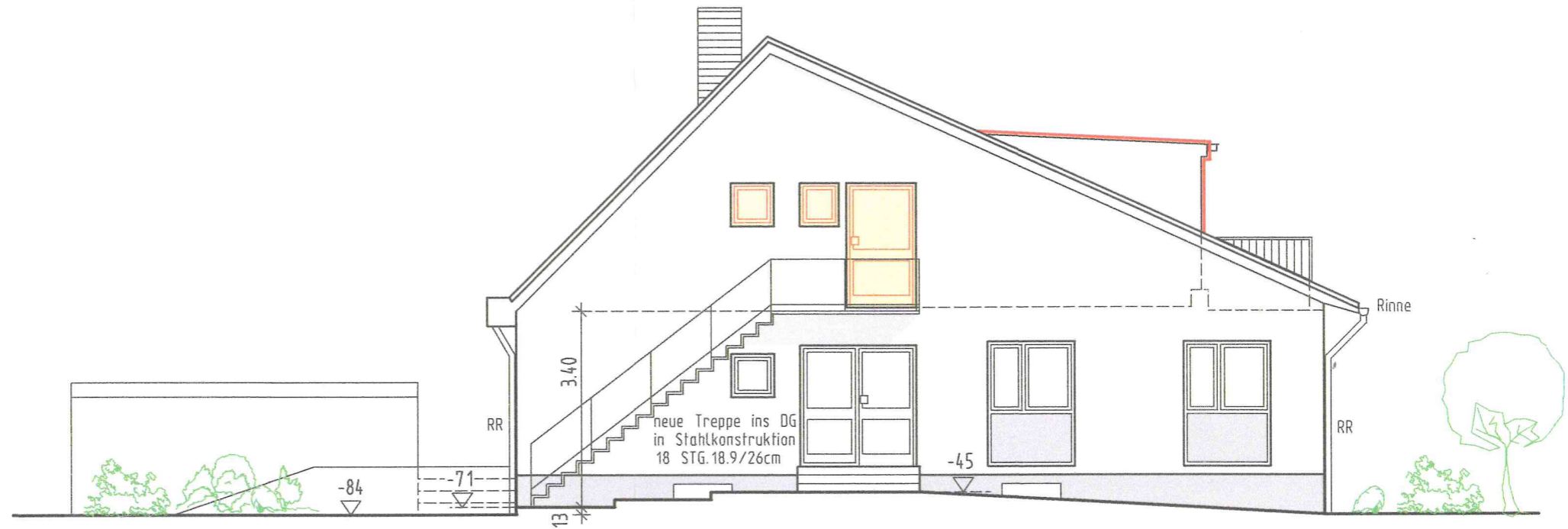
Ost - Ansicht M 1 : 100
