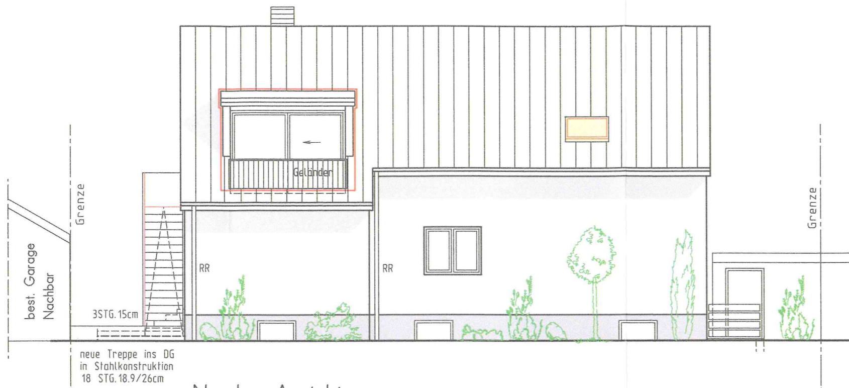
Nord - Ansicht M 1 : 100
