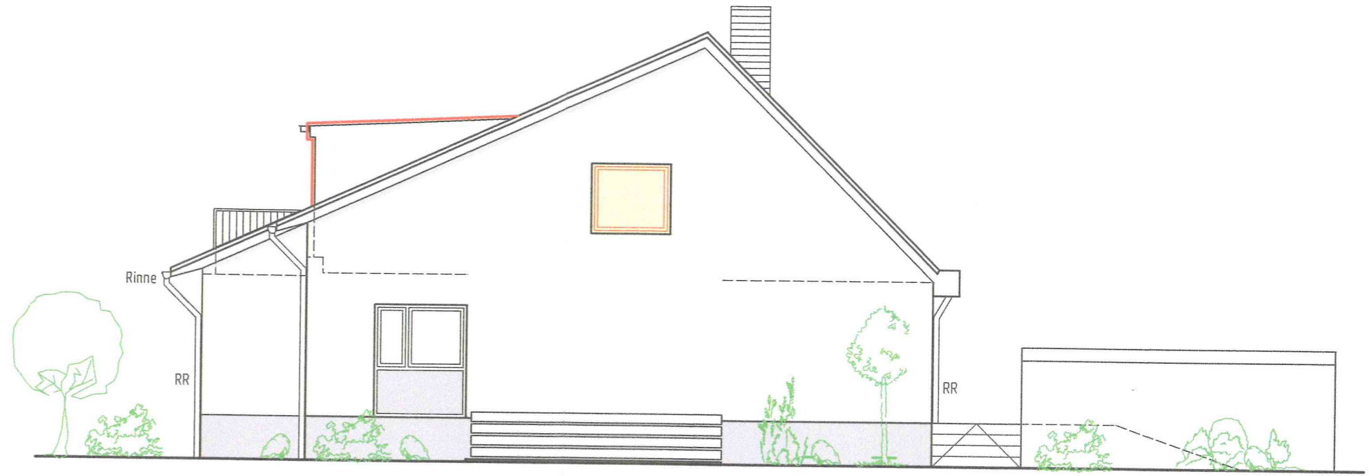
West - Ansicht M 1 : 100
