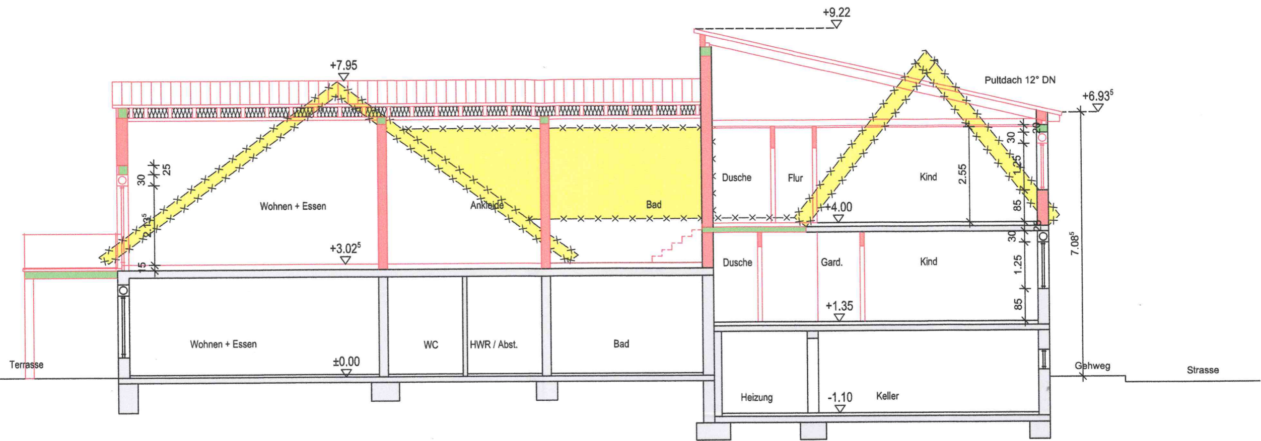
Schnitt A-A
