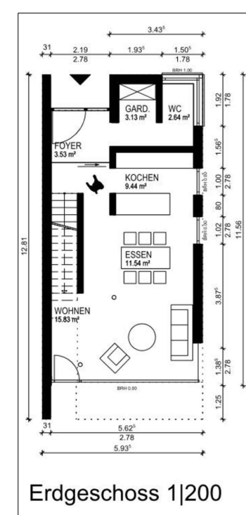
Grundrisse Reihenhäuser/Doppelhäuser M1:200
