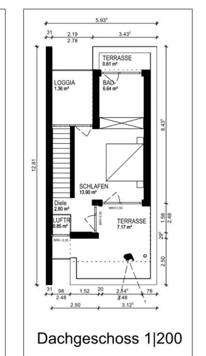
Grundrisse Reihenhäuser/Doppelhäuser M1:200
