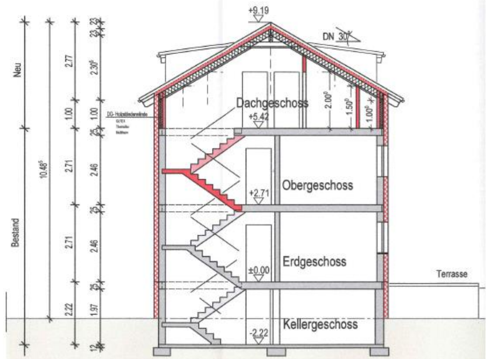
SCHNITT A-A
