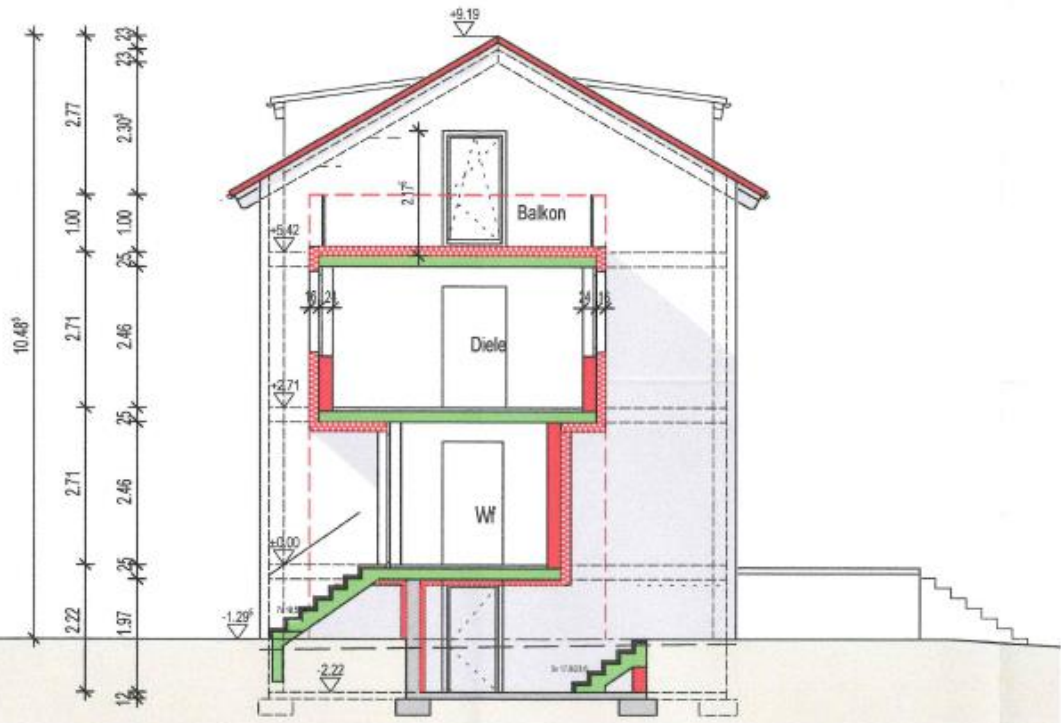
SCHNITT B-B
