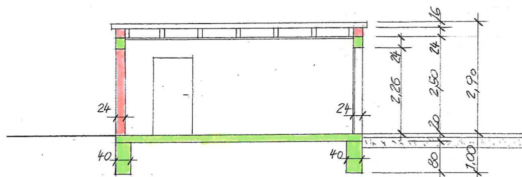
SCHNITT A-A
