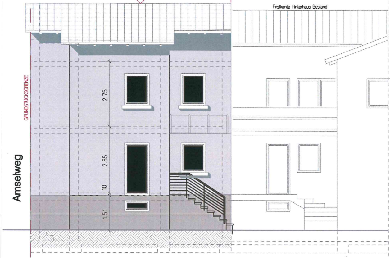
Nordseite M.1:100 Höhenbezug Vermesser Firsthöhe 19.55 NEU BESTAND
