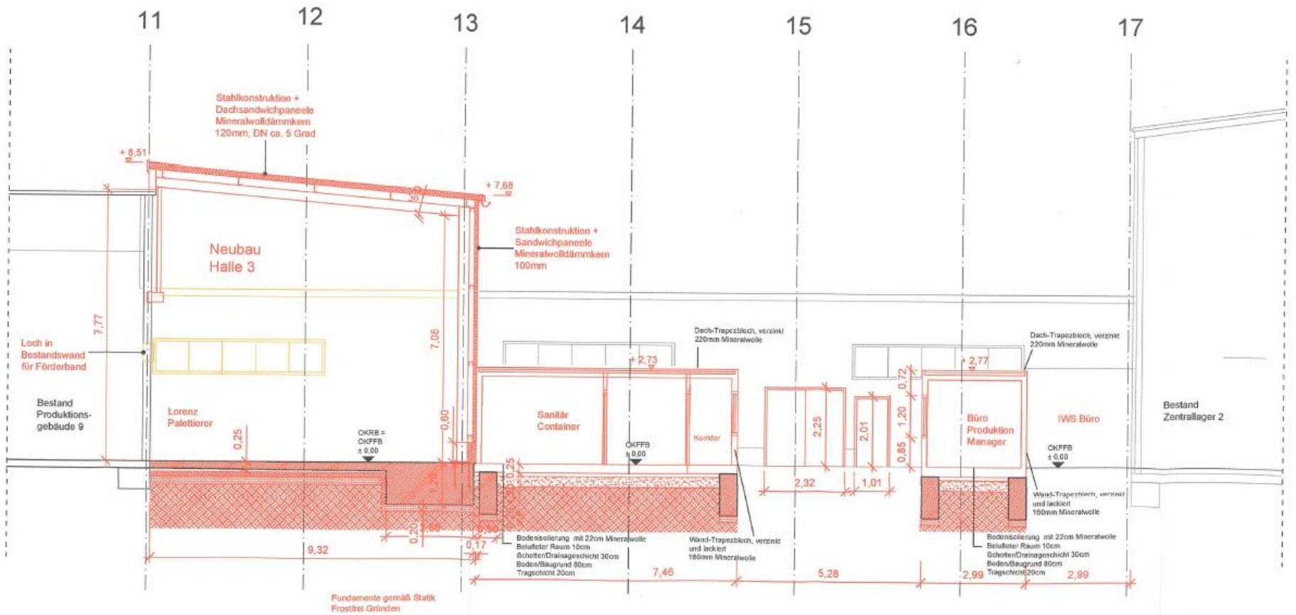
Halle 3 - Schnitt L-L
