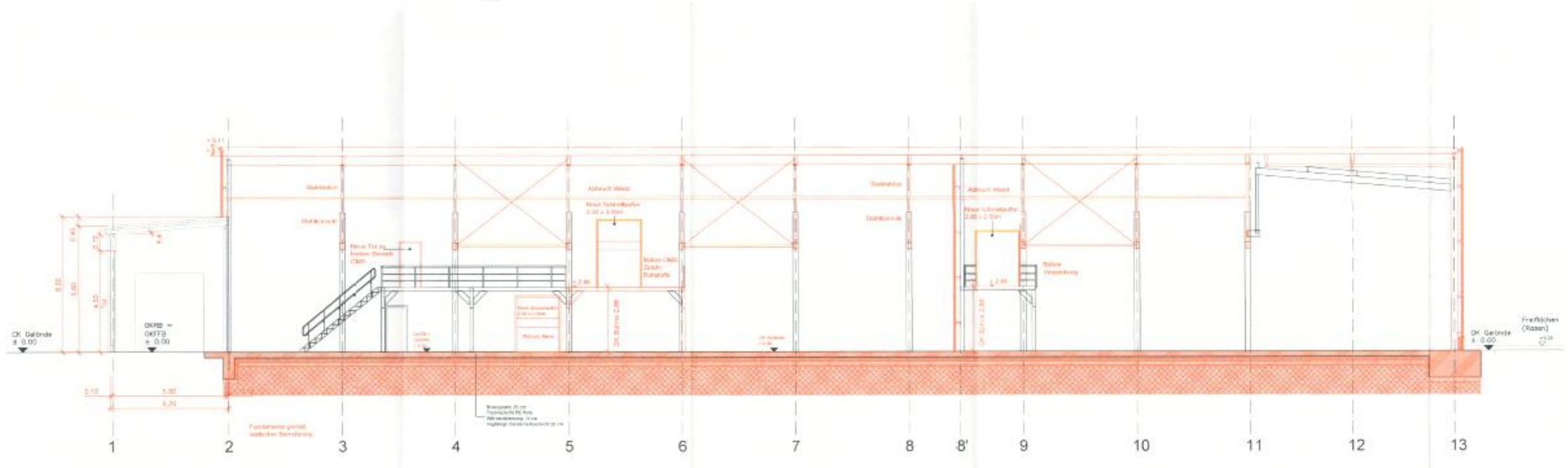
Halle 3 - Schnitt I-I
