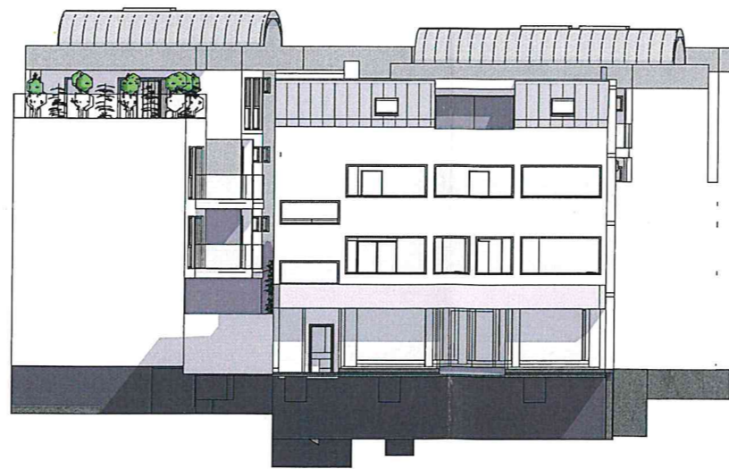
ANSICHT OST
