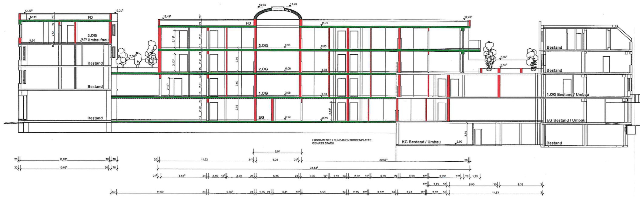
SCHNITT 1
