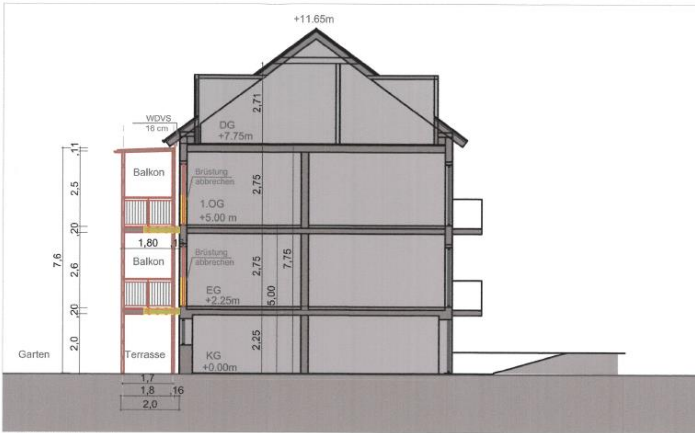
SCHNITT A-A
