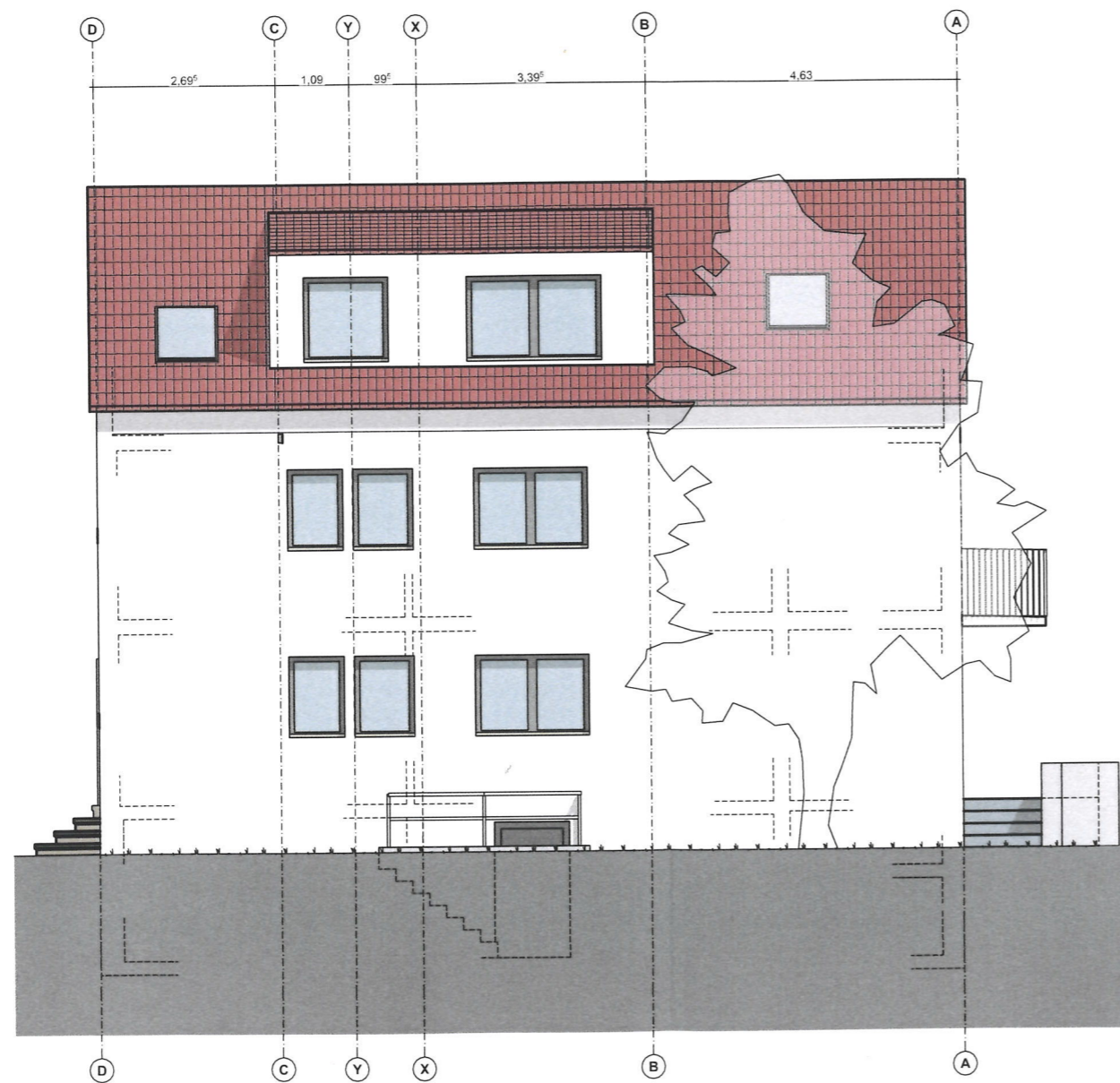
ANSICHT NORD M 1:100 GARTENSEITE
