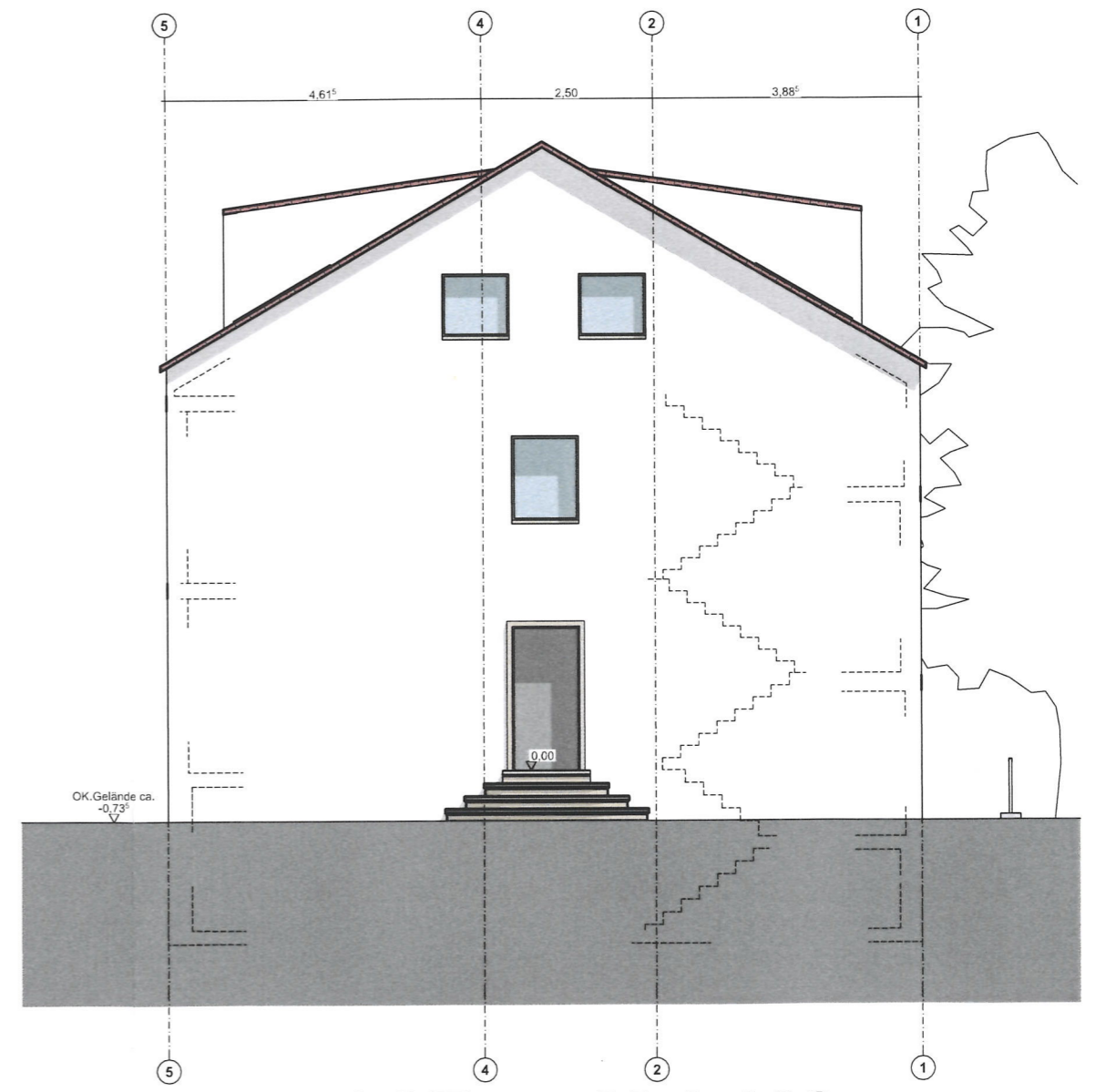
ANSICHT OST M 1:100
