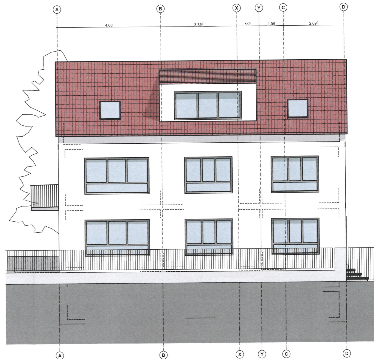
ANSICHT SÜD M 1:100 STRASSESEITE
