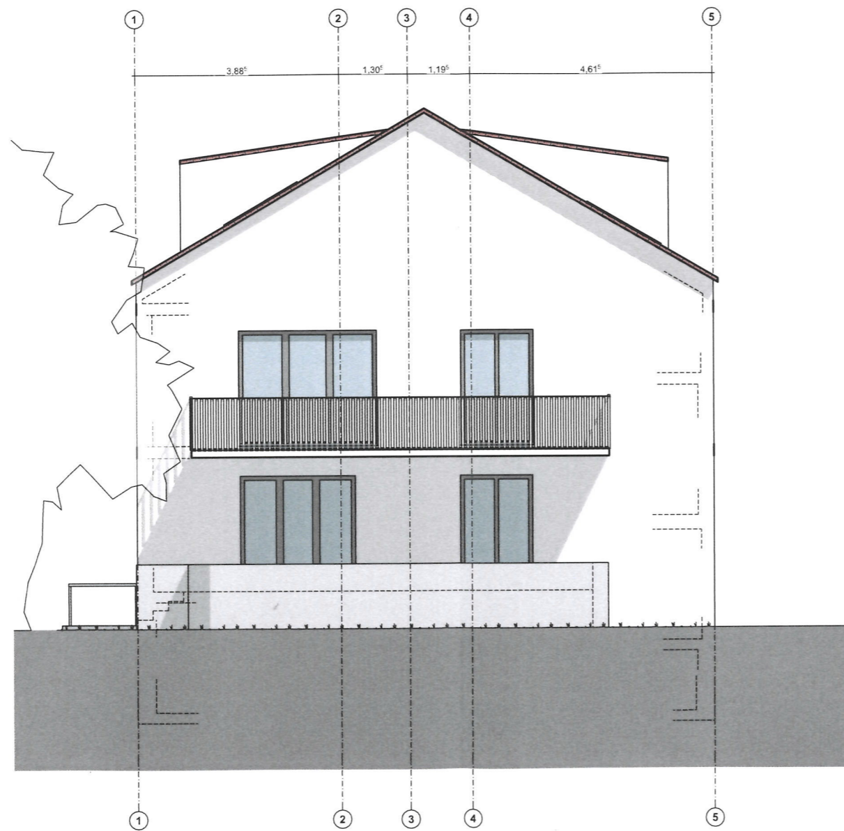
ANSICHT WEST M 1:100
