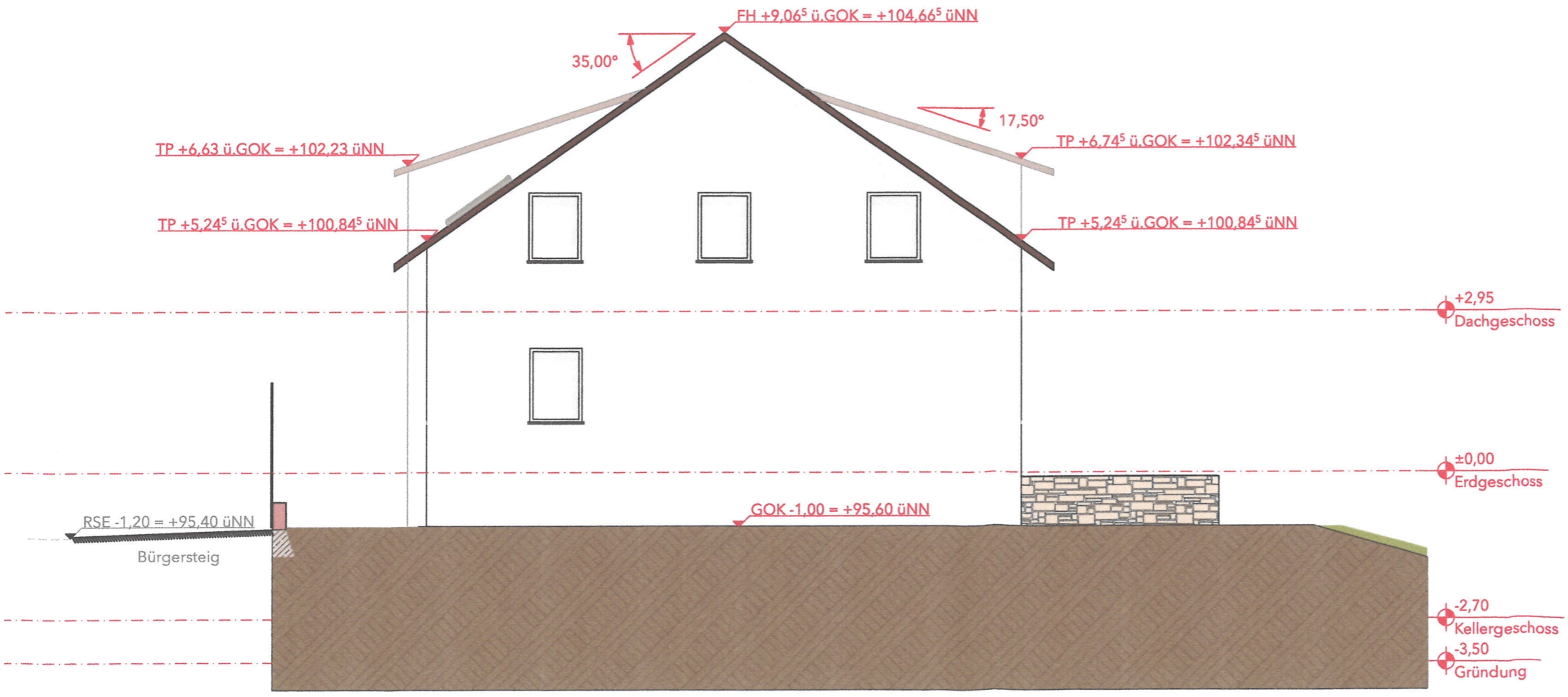
A-04 Ansicht Westen
