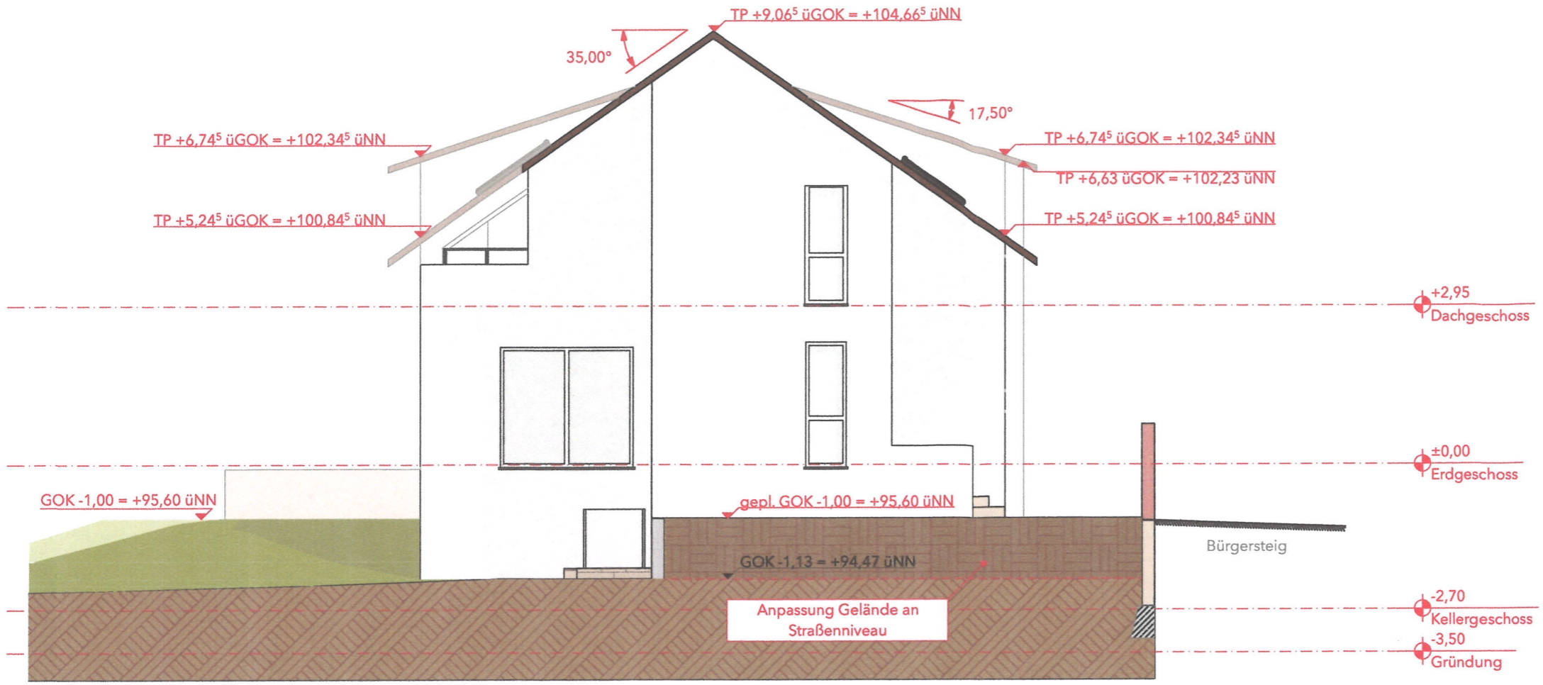
A-03 Ansicht Osten
