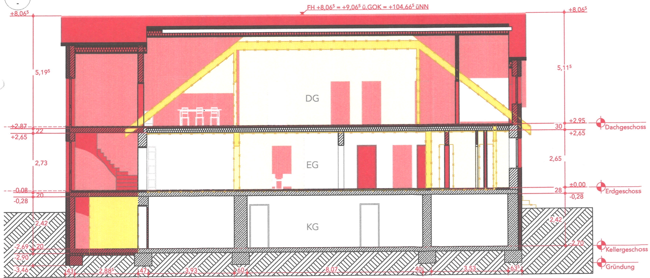
S-02 Schnitt B-B
