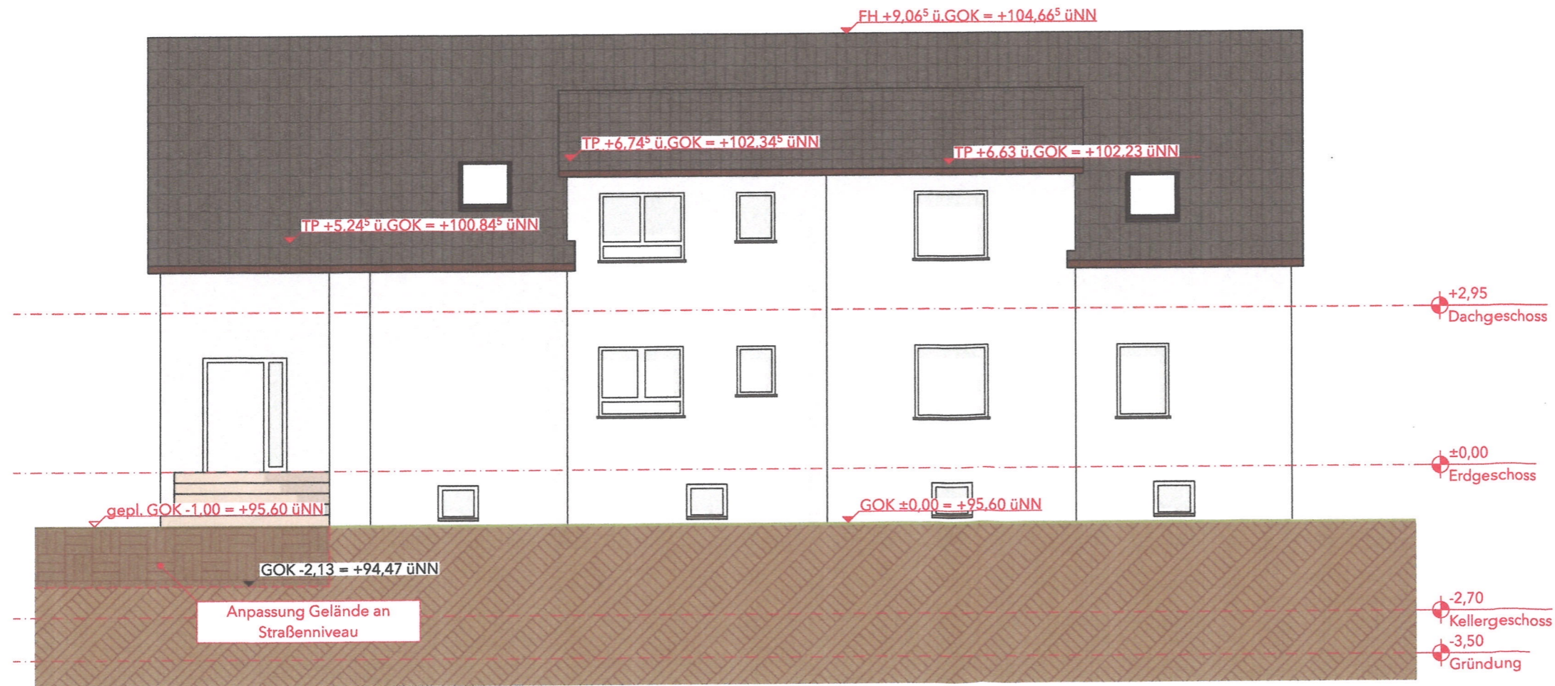
A-01 Ansicht Süden
