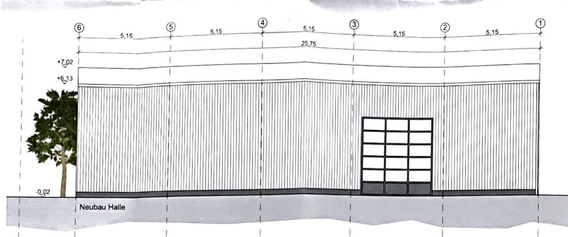
Ansicht Nord M 1:100
