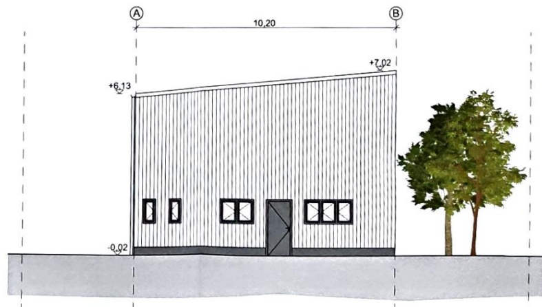
Ansicht West M 1:100
