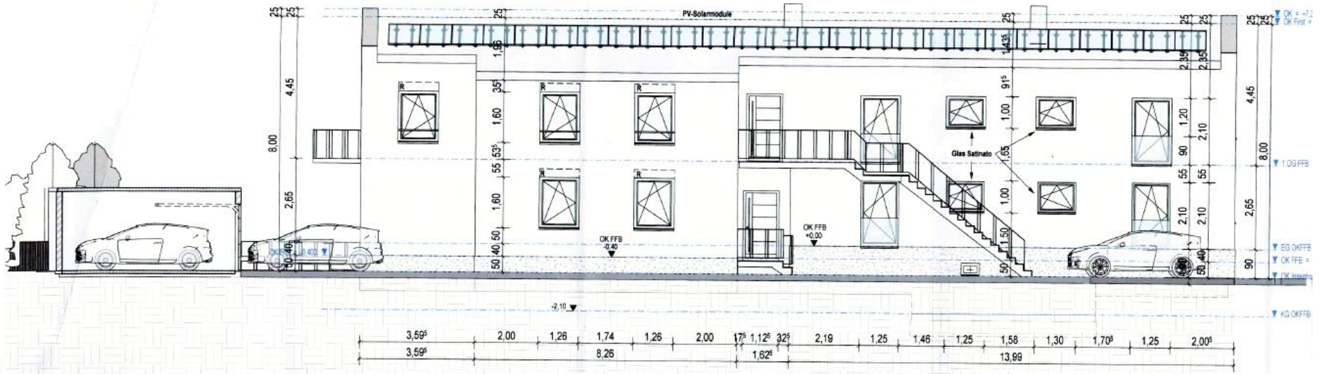
Ansicht Süd
