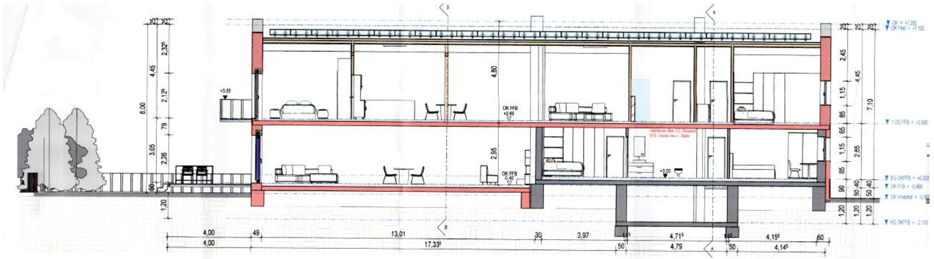
Schnitt 2-2
