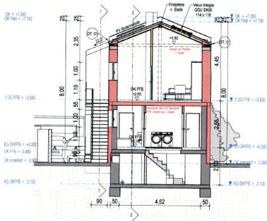
Schnitt A-A
