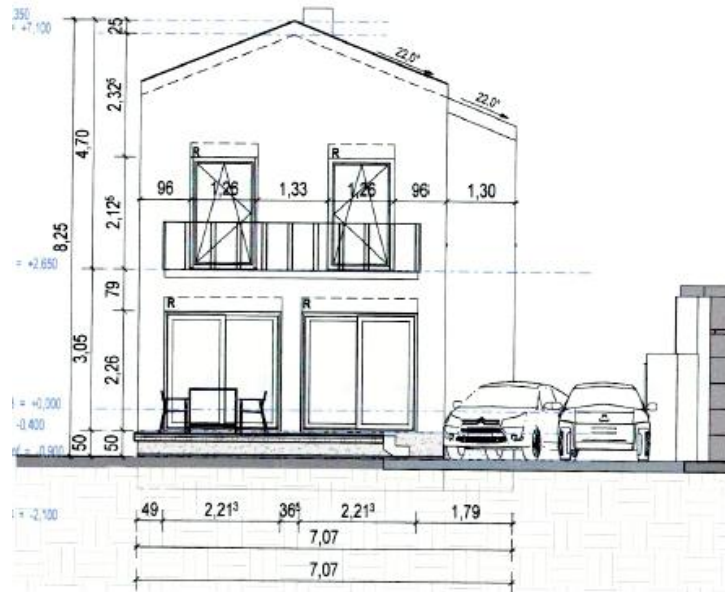
Ansicht West
