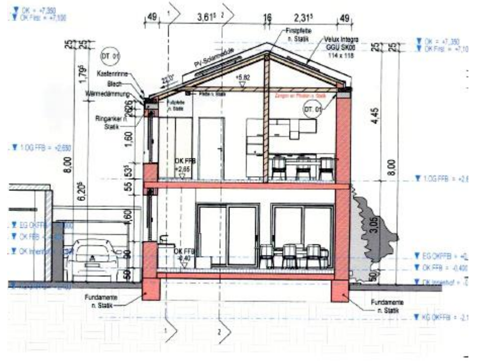
Schnitt B-B
