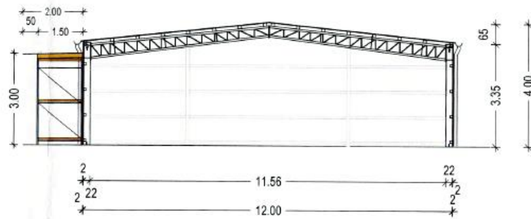
Schnitt A-A
