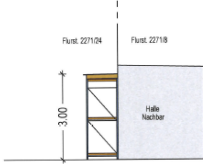
Ansicht Ost
