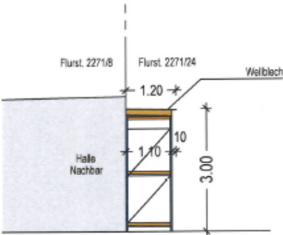
Ansicht West
