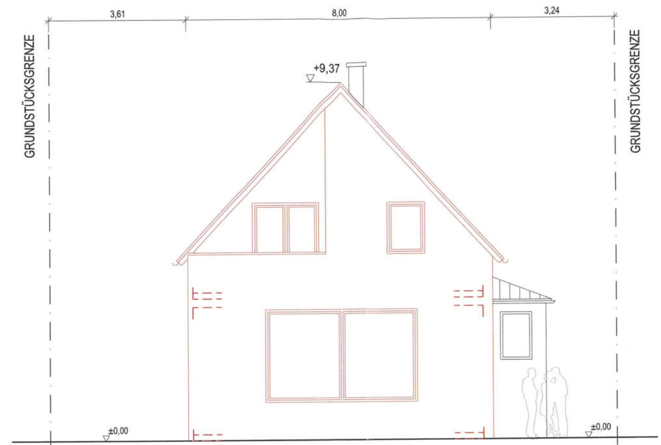
Ansicht Süden
