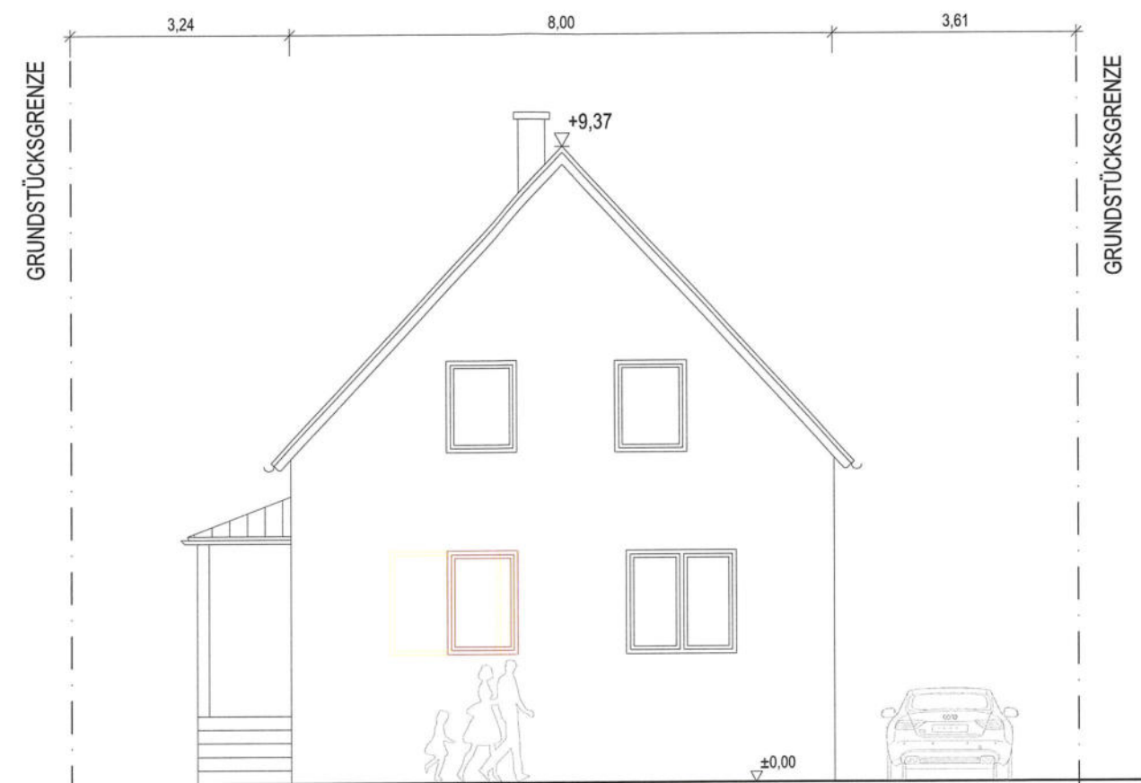
Ansicht Norden
