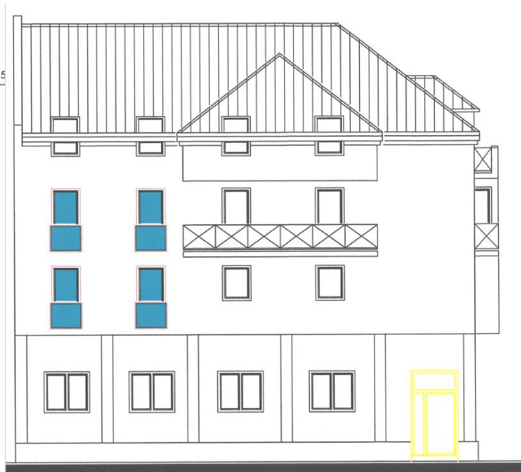
Ansicht West
