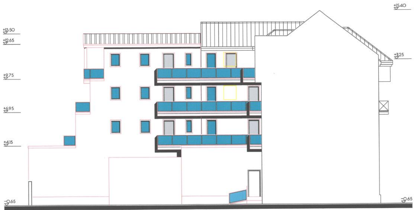
Ansicht Nord
