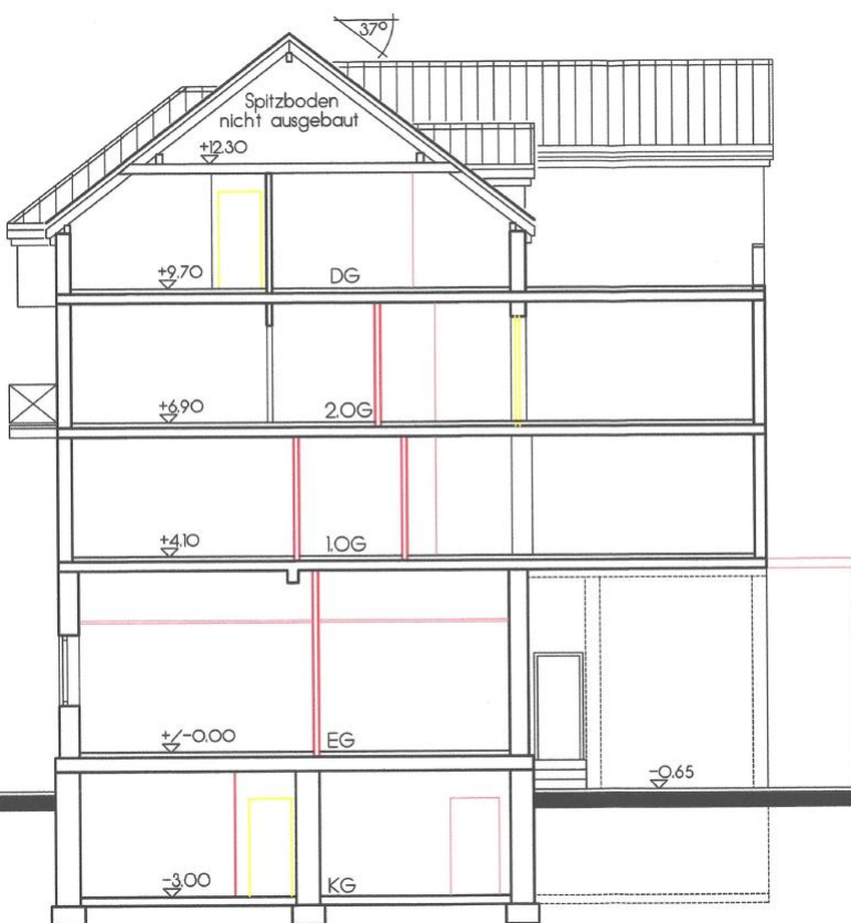
Schnitt Bestandsgebäude
