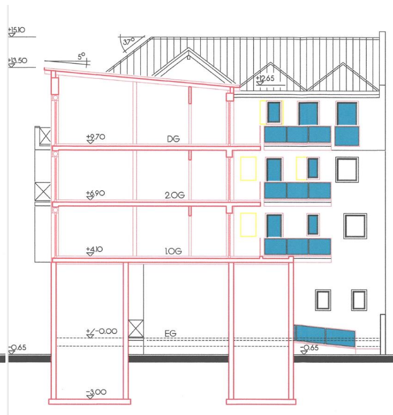
Schnitt Neubau/Ansicht Ost
