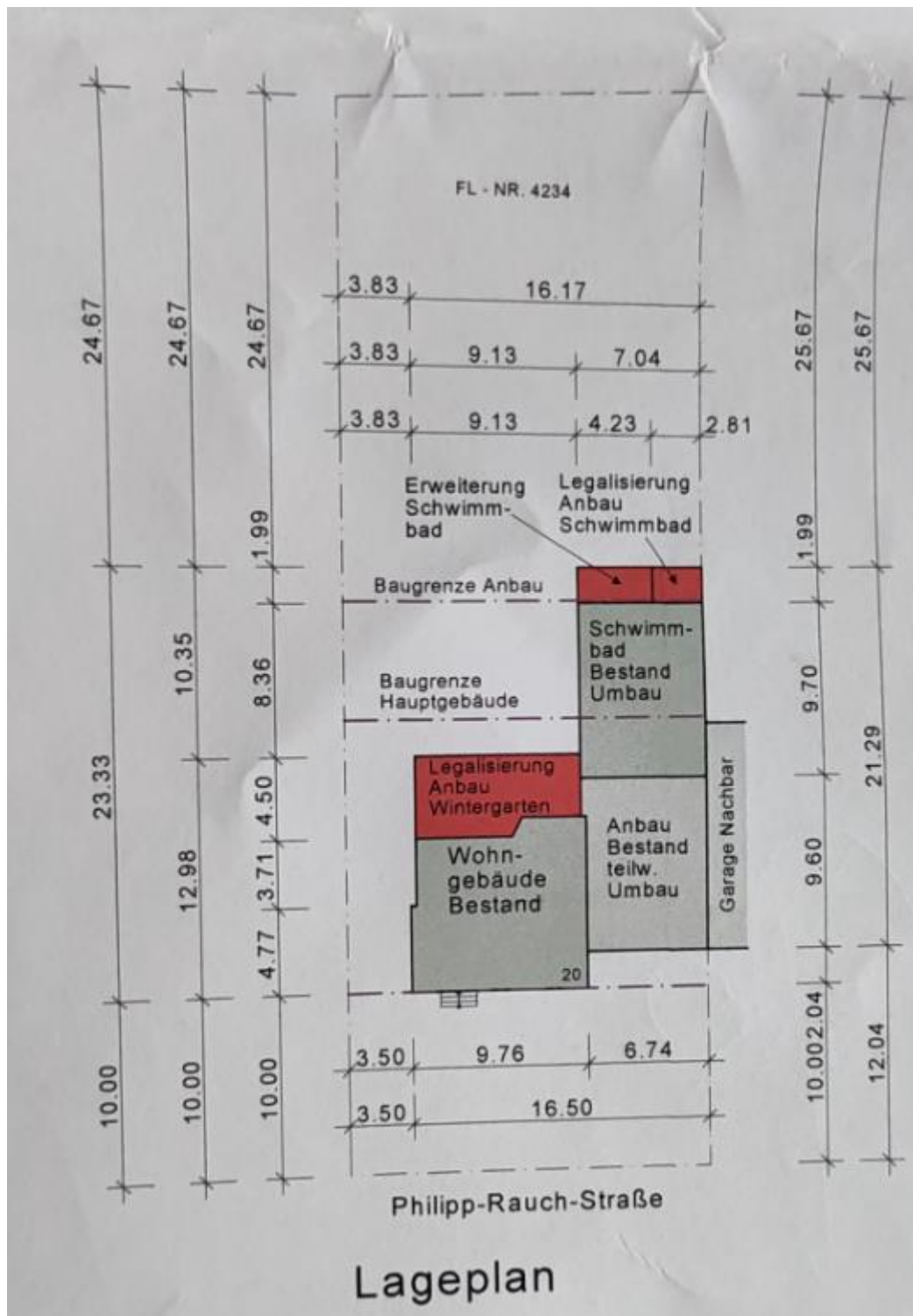
Abb. 4: Lageplan
