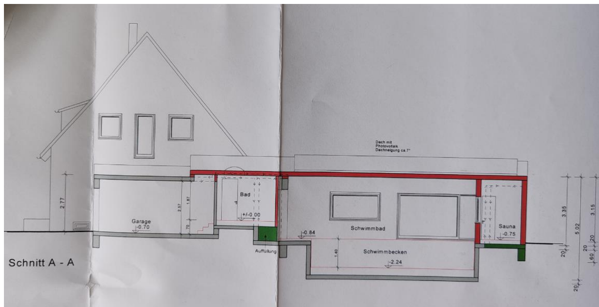
Abb. 5: Ansichten und Schnitte
