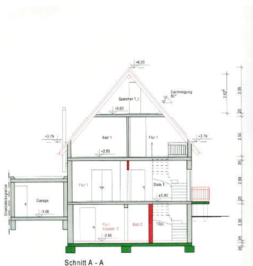
Abb. 6 Schnitte
