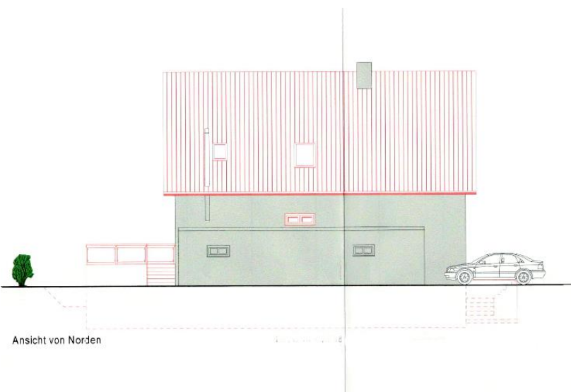
Abb. 5 Ansichten Nord und West
