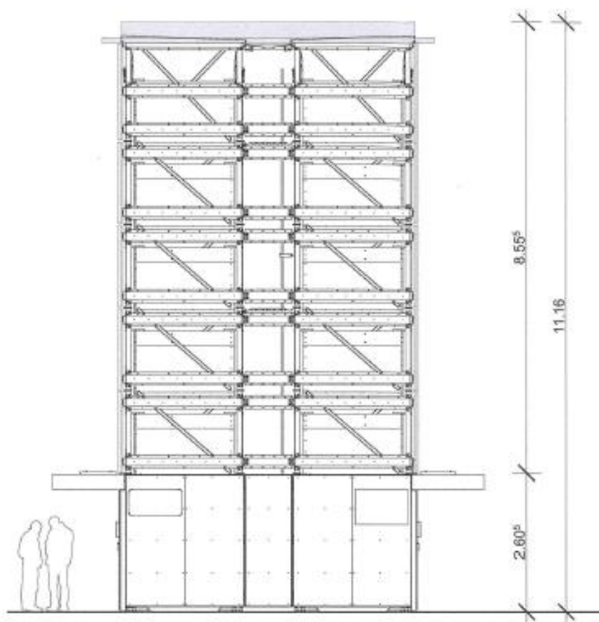
Schnitt A-A
