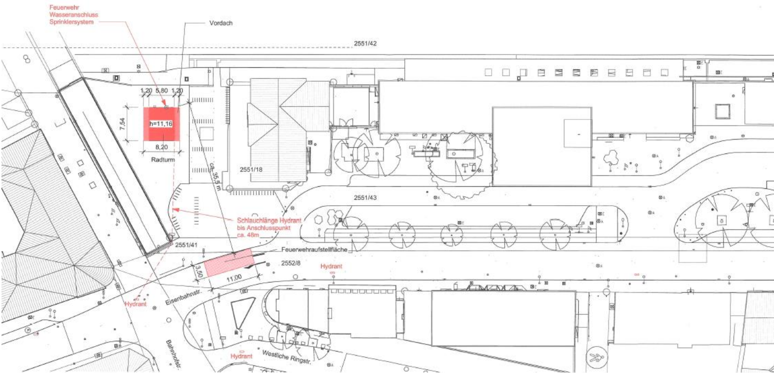
Abb. 4 Lageplan
