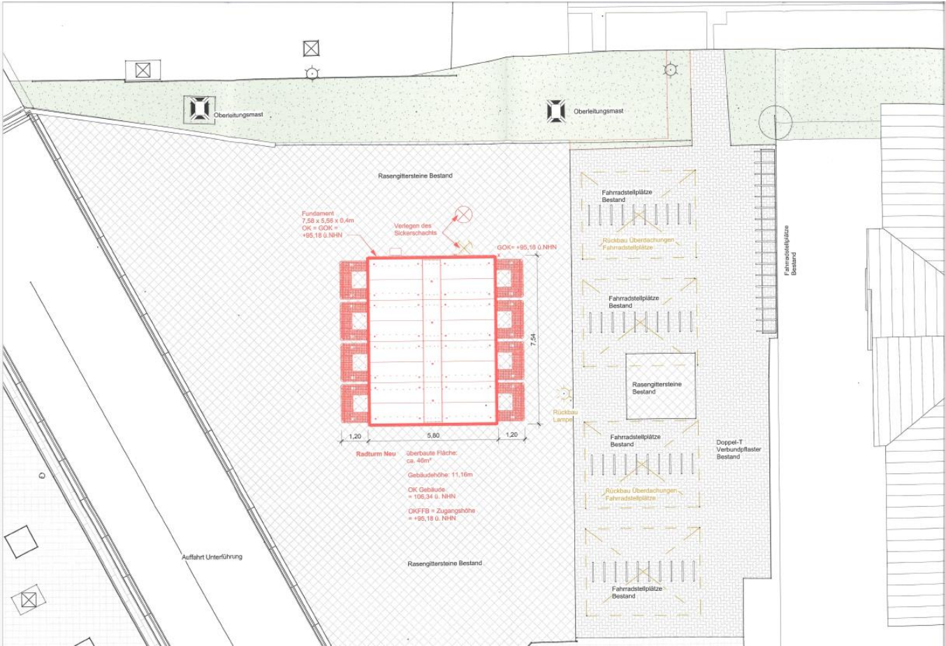
Abb. 5 Lageplan Freiflächen
