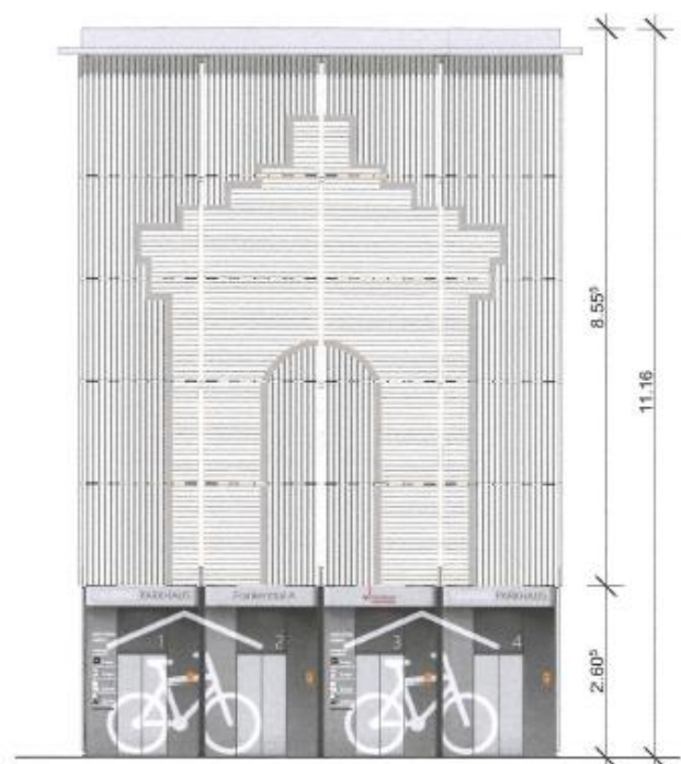
Ansicht NORD
