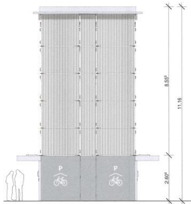
Ansicht WEST
