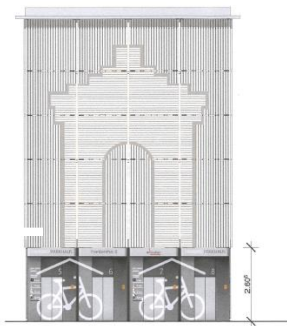
Ansicht SUD
