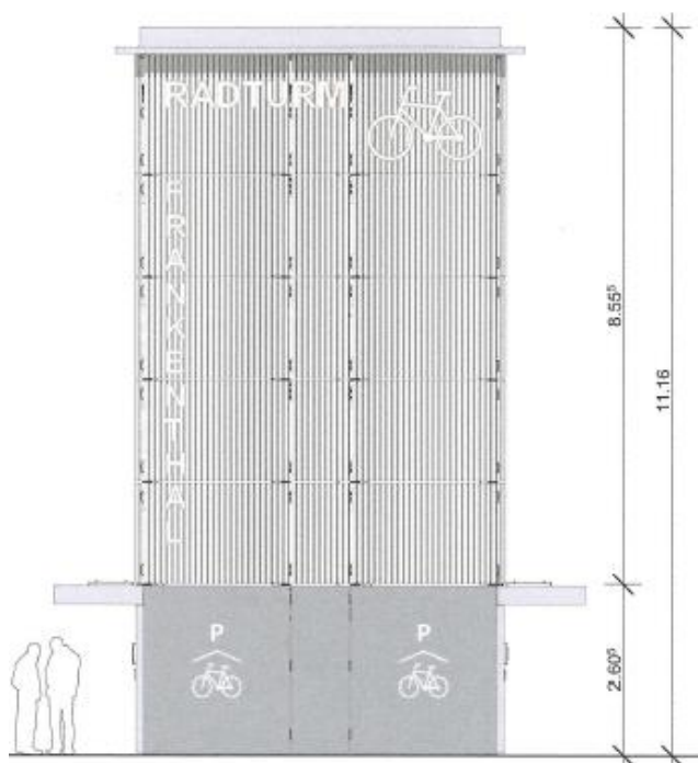
Ansicht OST
