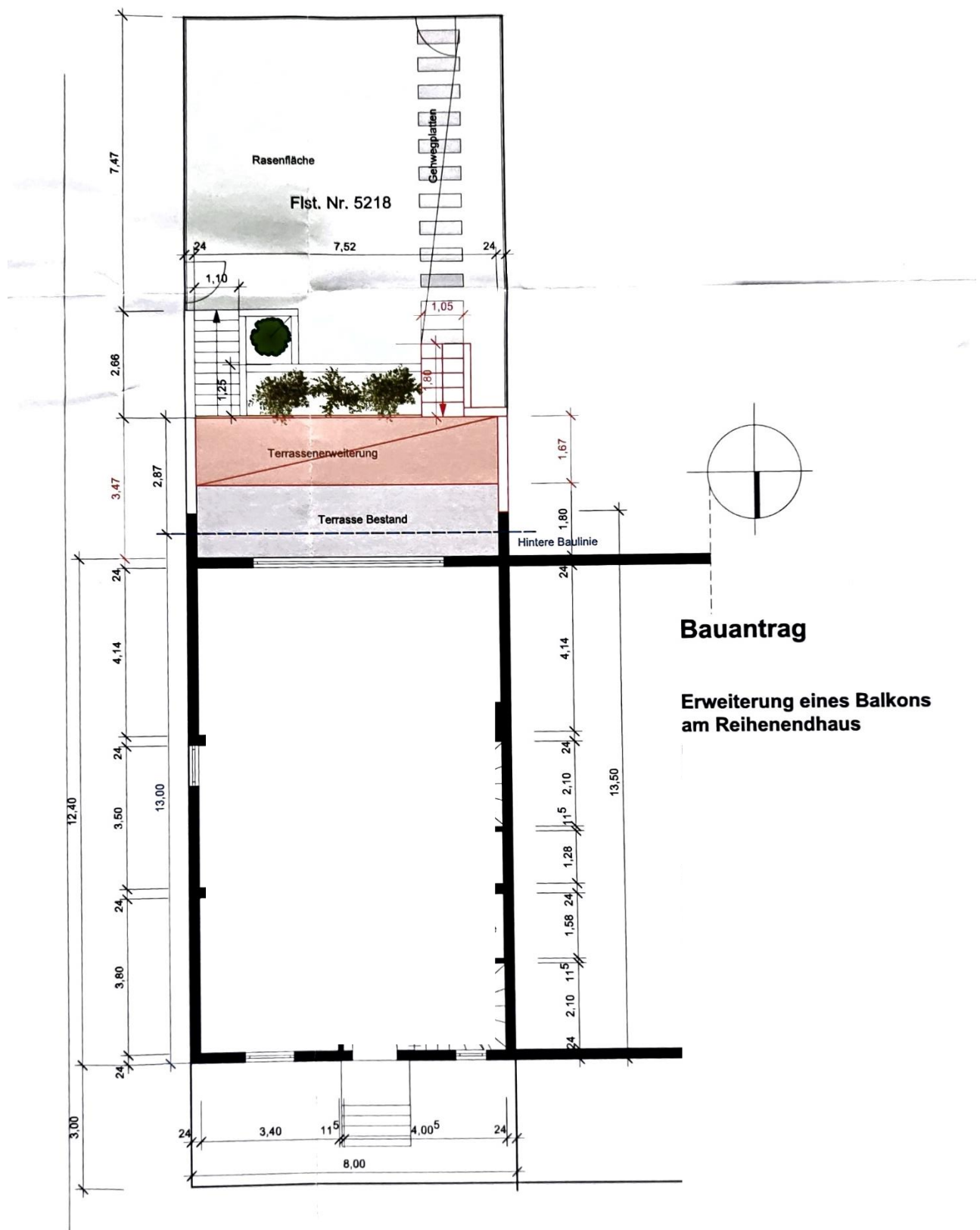
Abb. 5: Freiflächenplan
