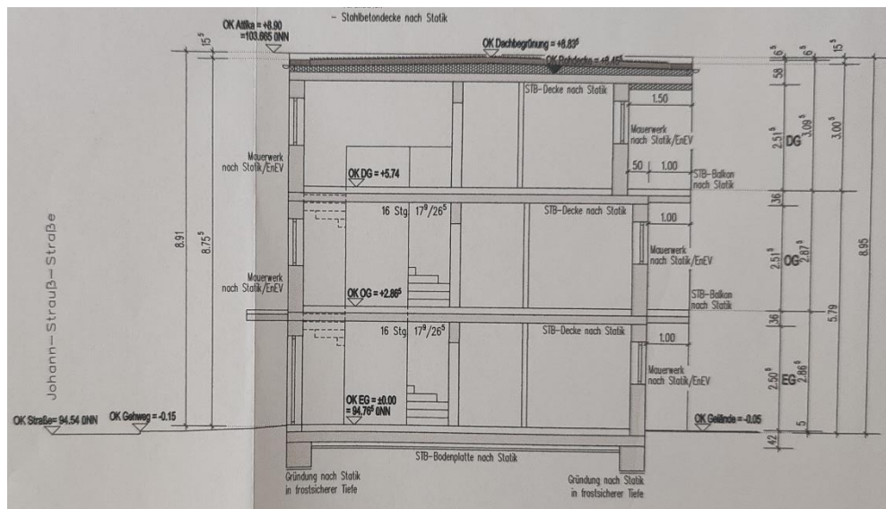
Abb. 5 Schnitt
