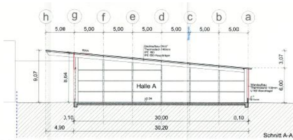
Abb. 4-5: Schnitte Halle A und Halle B
