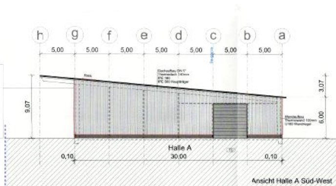
Abb. 7-9: Ansichten: Halle A und Halle B Süd-West, Halle A Nord-Ost
